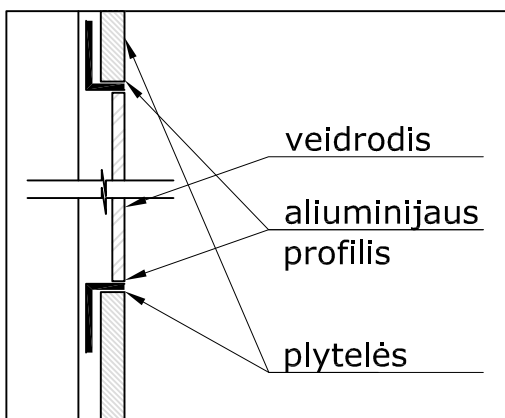
VEIDRODŽIO MONTAVIMO DETALĖ NR.1
