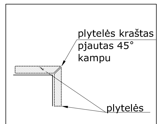
IŠORINIO KAMPO DETALĖ DETALĖ NR.3
